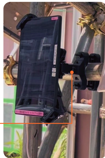
クランプ固定用治具
